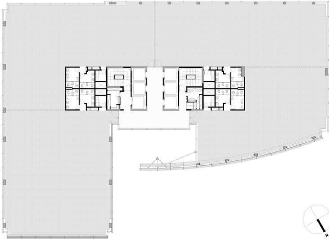
PLANTA TIPO
